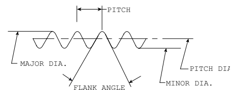
N.P.T. PIPE THREAD
