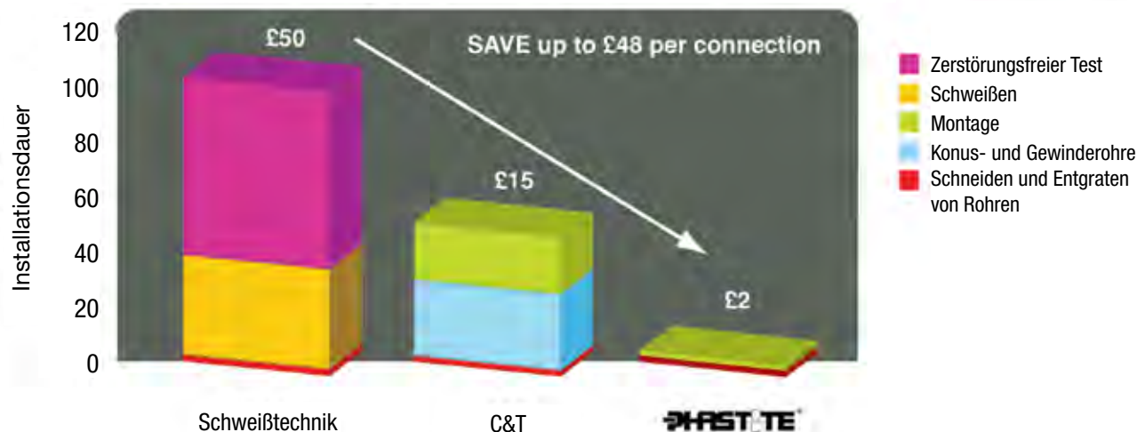
Ungefähre Einsparungen im Vergleich zu anderen Anschlussarten
