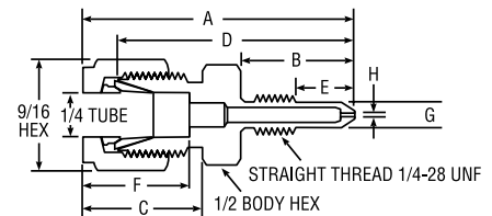
Kalibrierungsadapter für Honeywell DP Transmitter
